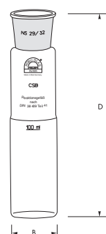
CSB-Reaktionsgefäß mit exaktem Durchmesser nach DIN 38409 CSB-Reaction vessel with exact diameter according to DIN 38409
