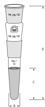
HCL-Absorber nach DIN 38409 für die CSB-Bestimmung HCL-Absorber for determination of O 2 -demand in water 1 mol K 2 Cr 2 O 7 = 1.5 mol O 2 DIN 38409
