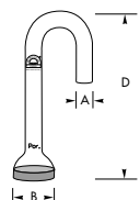
Mikro-Eintauchfilter für umgekehrte Filtration, Rohr gebogen Micro-immersion filters for reverse filtration, bent tube
