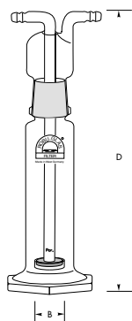
Gaswaschflaschen Aufsatz mit Filterplatte, Normschliff Gas washing bottles Head with fritted disc, standard taper joint
