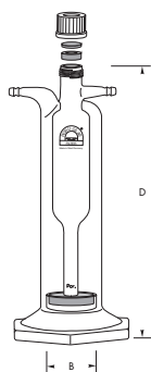
Gaswaschflasche mit Überdrucksicherung Gas washing bottle with overpressure safety foil
