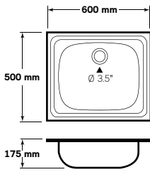
AV 060 MB, MB/C
