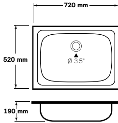
AV 720 MB, MB/C
