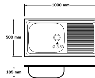
AV 100 MB, MB/C
