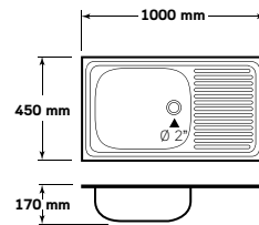
AVP 075 MA, MA/C
