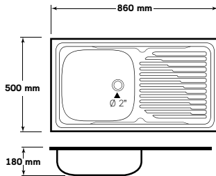
AV 5086 MA, MA/C
