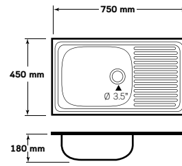
AV 075 MB, MB/C
