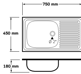
AV 075 MA, MA/C
