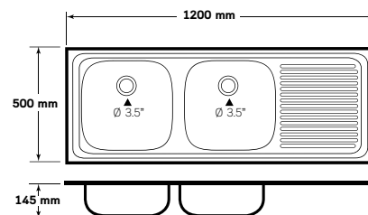
AV 140 MB, MB/C
