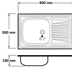
AV 080 MA, MA/C
