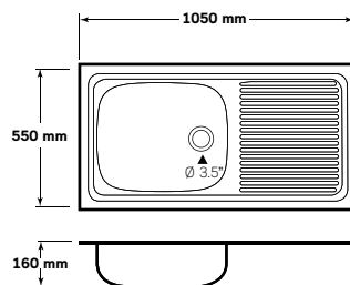
AV 105 MB, MB/C
