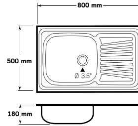
AV 080 MB, MB/C
