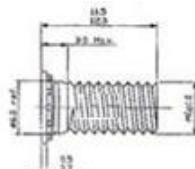
สกรูฟาสเทนนิ่ง (ซุบรู้ง) (FASTENING BOLT PFH ST5.6)
