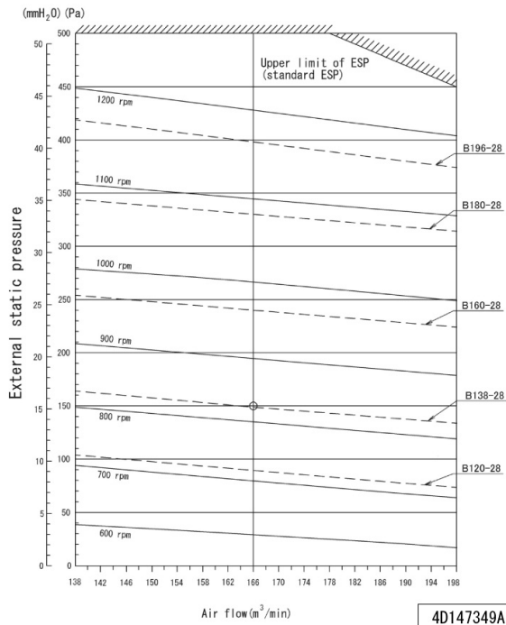
FVPR18QY2S FVPR20QY2S
