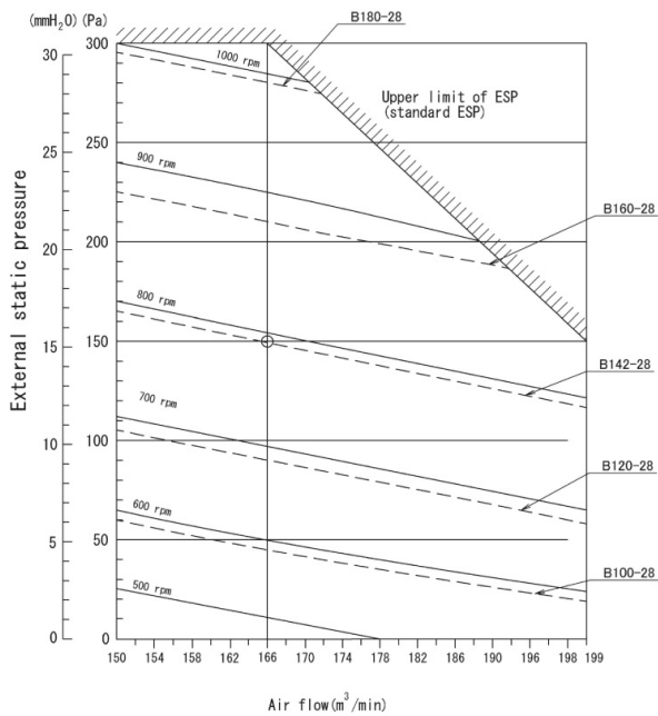
FDR18QY2S FDR20QY2S
