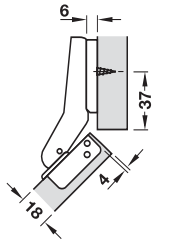
Distance 6 mm, half overlay ระยะห่าง 6 มม., กลางขอบ
