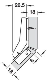
Distance 4 mm, mitre ระยะห่าง 4 มม.
