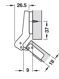
Mounting plate distance ขนาดฐานรองบานพับ
