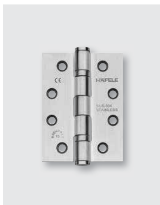
สแตนเลสสตีลด้าน
