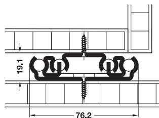
Base mounted รับใต้
