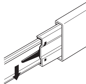
Disengaging การปลดรางลิ้นชัก
