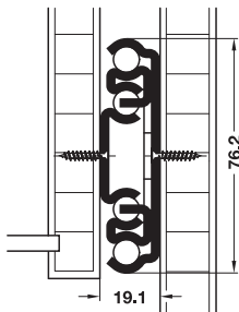
Side mounted รับข้าง
