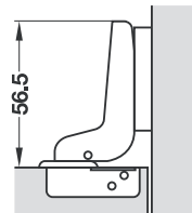
Inset แบบในขอบ
