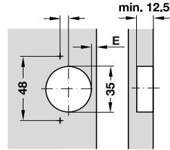
Drilling dimension for cup fixing ขนาดรูเจาะสำหรับถ้วยบานพับ
