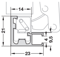
Groove shape รูปร่างของร่อง
