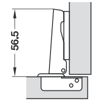
Full overlay แบบทับขอบ
