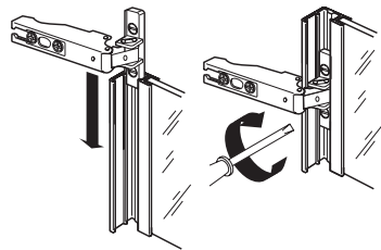
Installation การติดตั้ง
