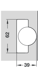
Cup dimension ขนาดถ้วยบานพับ
