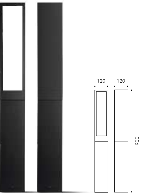
Microkuba long bollard H 900mm
