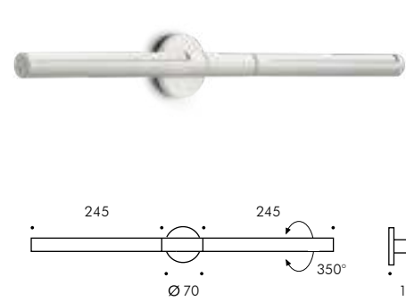
Spillo double applique
