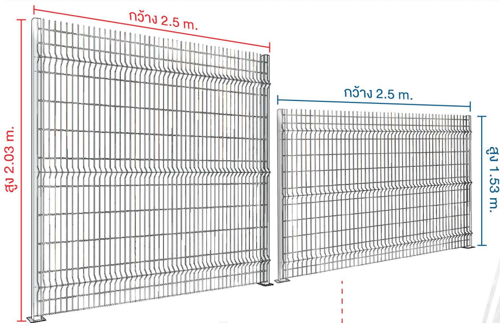
ขนาดแผงรั้ว ต่างกันที่ความสูง
