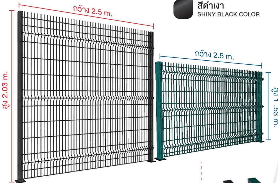
ขนาดแผงรั้ว ต่างกันที่ความสูง
