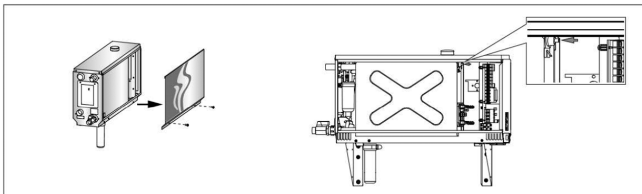
รูปที่ 14 การรีเซ็ตค่าตัวป้องกันความร้อนสูงเกินไป
