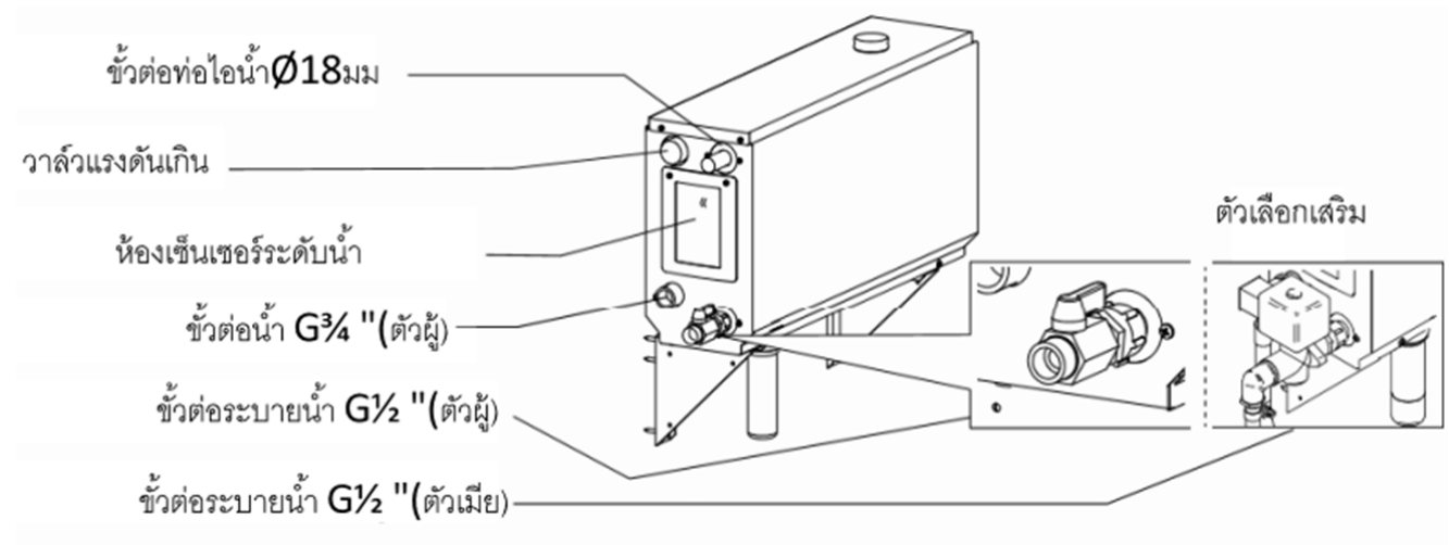
รูปที่ 8 การเชื่อมต่อเครื่องกำเนิดไอน้ำ
