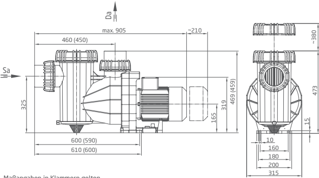
Maßangaben in Klammern gelten für BADU Resort 30 bis BADU Resort 45.
