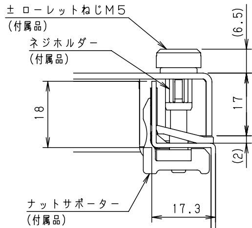
A部断面詳細(1:1)
