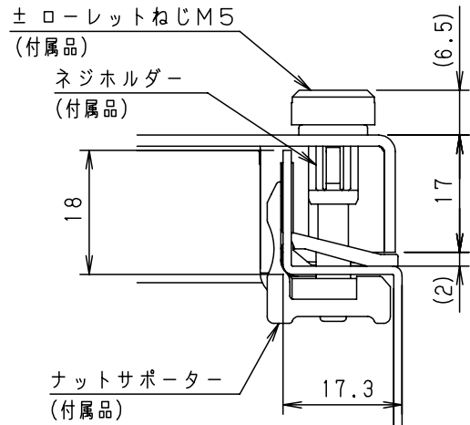
A部断面詳細 (1:1)
