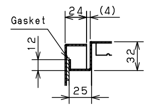
CROSS SECTION A-A 1:3
