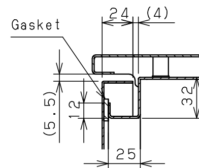
CROSS SECTION A-A 1 : 3
