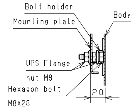
CROSS SECTION B-B 1 : 3
