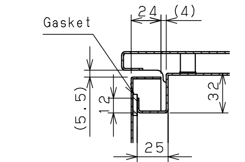
CROSS SECTION A-A 1 : 3
