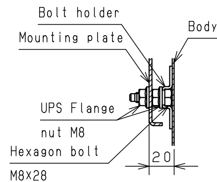
CROSS SECTION B-B 1 : 3
