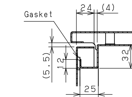
CROSS SECTION A-A 1 : 3
