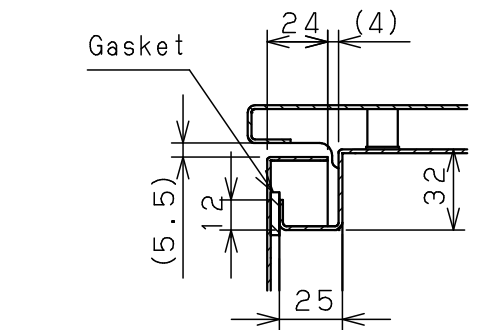
CROSS SECTION A-A 1 : 3
