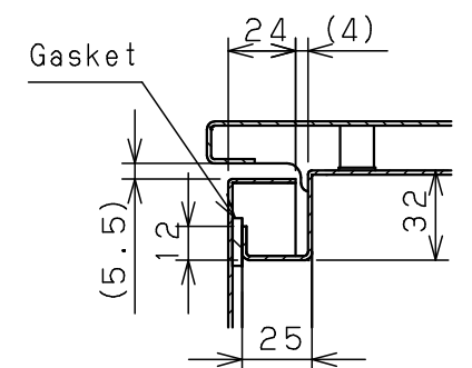
CROSS SECTION A-A 1 : 3
