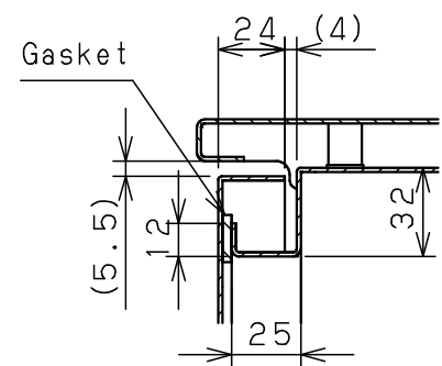
CROSS SECTION A-A 1 : 3
