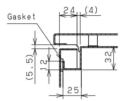
CROSS SECTION A-A 1 : 3
