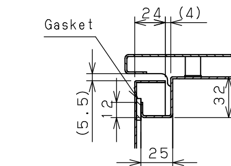
CROSS SECTION A-A 1 : 3
