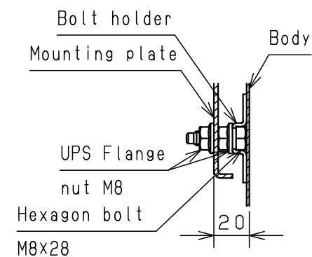
CROSS SECTION B-B 1 : 3
