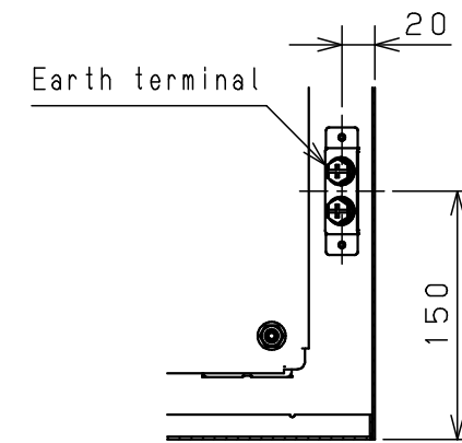
CROSS SECTION C-C 1 : 5
