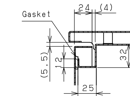
CROSS SECTION A-A 1 : 3
