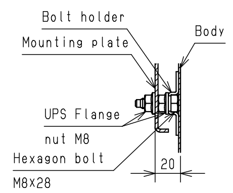
CROSS SECTION B-B 1 : 3
