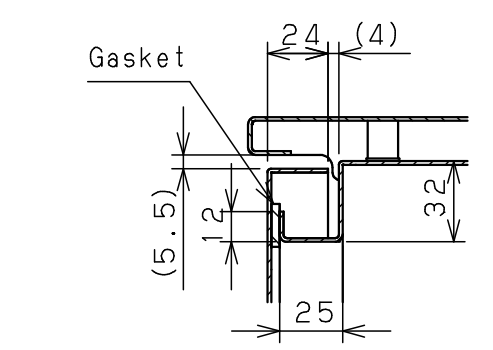
CROSS SECTION A-A 1 : 3
