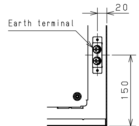
CROSS SECTION C-C 1 : 5
