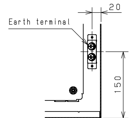
CROSS SECTION C-C 1 : 5
