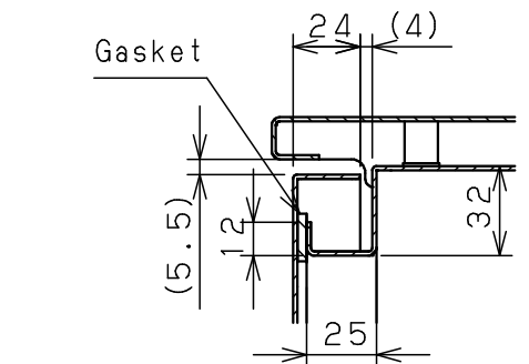
CROSS SECTION A-A 1 : 3
