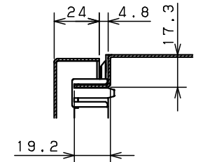
CROSS SECTION A-A 1:2
