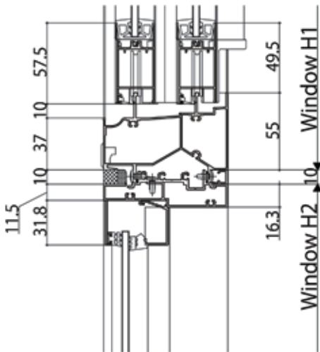
Transom A
