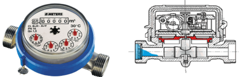
รูปที่ 1-13 มาตรใบพัดแบบช่องรับน้ำช่องเดียว (Single- Jet Meters)
