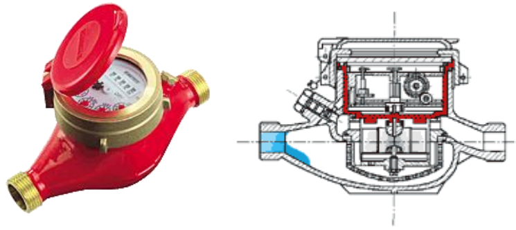
รูปที่ 1-14 มาตรใบพัดแบบช่องรับน้ำหลายช่อง (Multi- Jet Meters)
