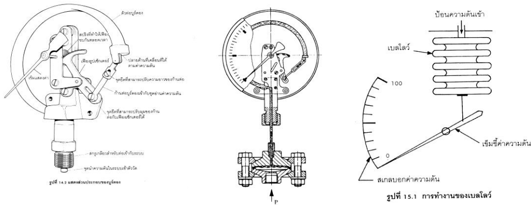
รูปที่ 1-18 เกจวัดความดันแบบต่าง ๆ
