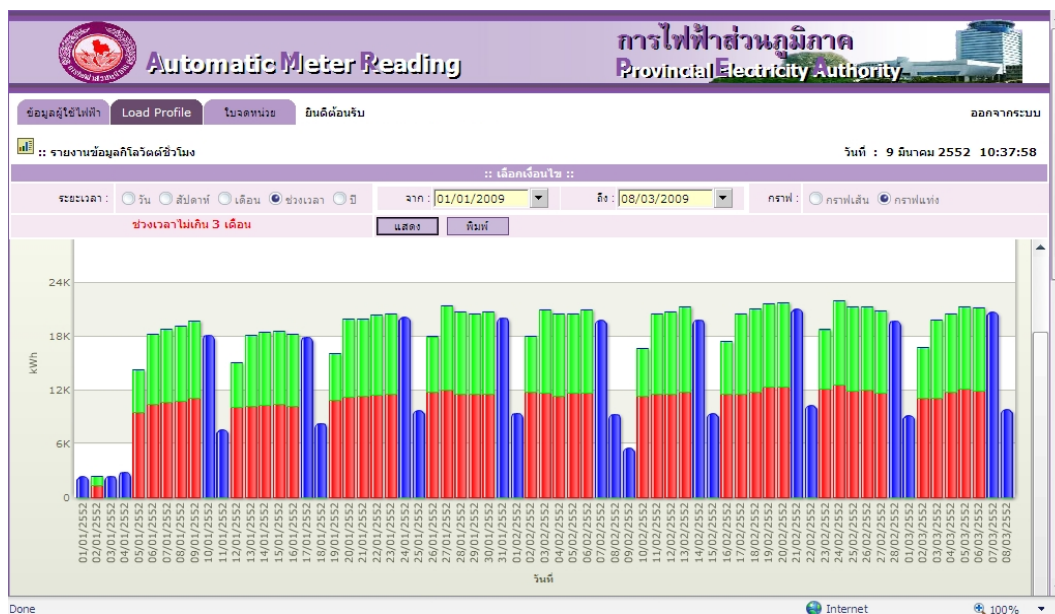
รูปที่ 2-36 แสดงหน่วยใช้ไฟฟ้า (kWh) ผ่านระบบ AMR ของผู้ใช้ไฟฟ้ายาวหนึ่ง
