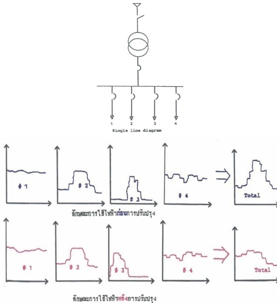
รูปที่ 2-35 แสดงการลดค่าความต้องการพลังไฟฟ้าสูงสุดด้วยการย้ายเวลาการทำงาน
