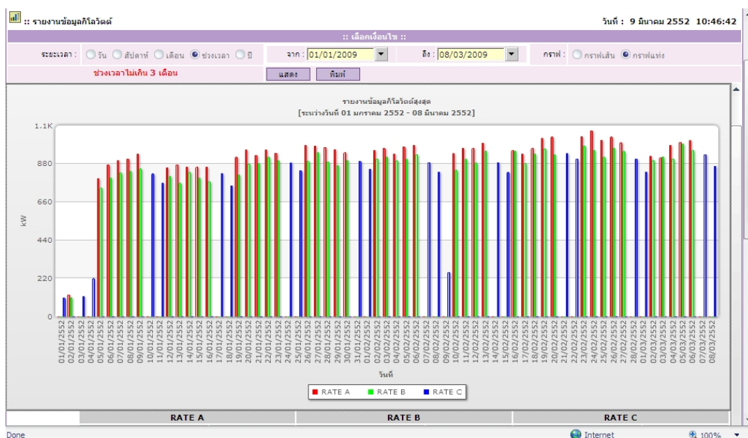
รูปที่ 2-37 ความต้องการพลังไฟฟ้าสูงสุดผ่านระบบ AMR ของผู้ใช้ไฟฟ้ายาวหนึ่ง
