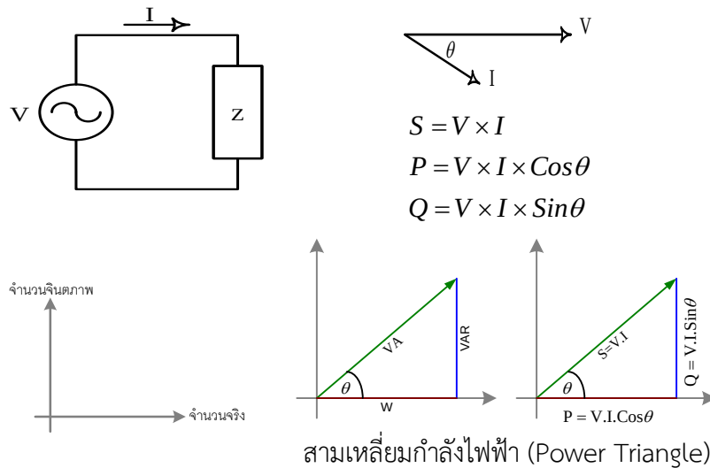
รูปที่ 2-12 สมการคำนวณกำลังไฟฟ้าและสามเหลี่ยมกำลังไฟฟ้า
