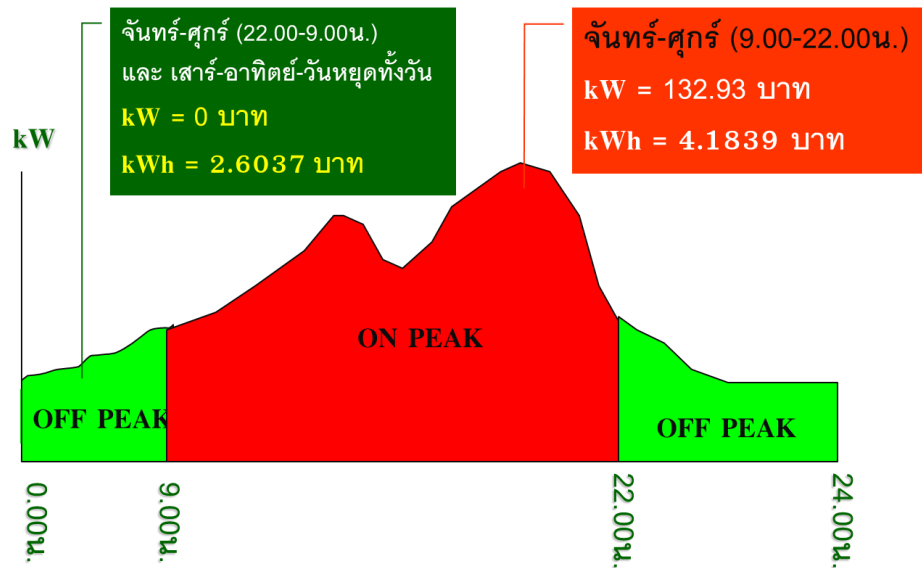
รูปที่ 2-24 การแบ่งช่วงเวลาตามอัตรา TOU
