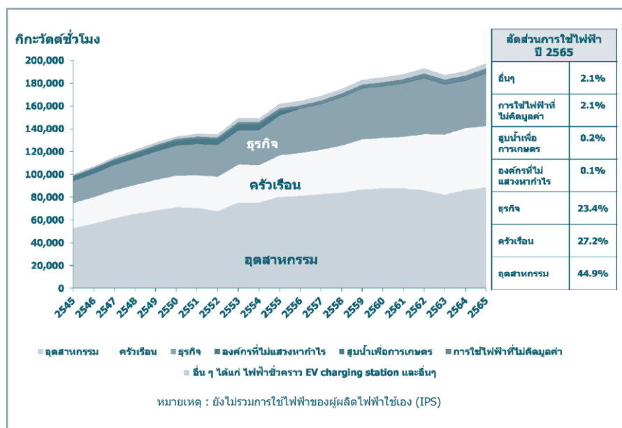
รูปที่ 1.2-17 การใช้ไฟฟ้ารายสาขา ปี 2565
