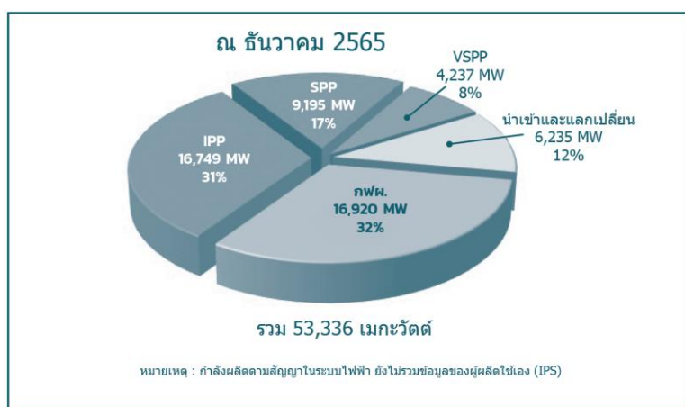
รูปที่ 1.2-15 กำลังการผลิตตามสัญญาในระบบไฟฟ้า ปี 2565
