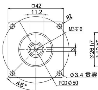
輸出端(output)
