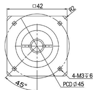
輸入端(input)
