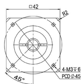
輸入端(input)
