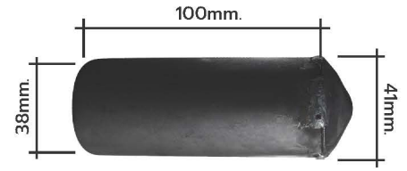
เมทัลโดเวลแคป Metal Dowel Cap
