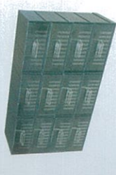
Model : 930/12 Ext. Size : 190 x 403 x 180 MM. Chs. Size : 190 x 125 x 40 MM. Chs. Q'ty : 12
