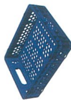
Model : DCT508 Ext. Size : 290 x 375 x 93 MM. Int. Size : 260 x 345 x 80 MM.
