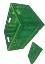
Model : 8002 Ext. Size : 404 x 602 x 231 MM. Int. Size : 364 x 565 x 222 MM.
