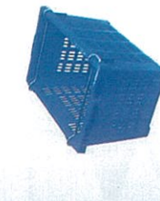
Model : 2542 Ext. Size : 365 x 590 x 325 MM. Int. Size : 325 x 528 x 310 MM.
