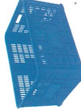
Model : 8070/2560 Ext. Size : 420 x 610 x 320 MM. Int. Size : 385 x 580 x 300 MM.
