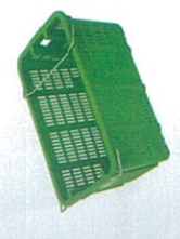
Model : 8203 Ext. Size : 430 x 700 x 290 MM. Int. Size : 385 x 580 x 235 MM.
