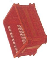
Model : 8241 Ext. Size : 338 x 442 x 237 MM. Int. Size : 308 x 400 x 232 MM.
