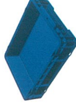
Model : DCT504 Ext. Size : 290 x 375 x 93 MM. Int. Size : 260 x 345 x 80 MM.
