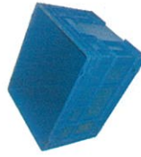
Model : DCT101 Ext. Size : 480 x 590 x 370 MM. Int. Size : 445 x 555 x 357 MM.
