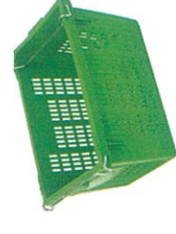
Model : 8202 Ext. Size : 370 x 580 x 340 MM. Int. Size : 325 x 526 x 323 MM.
