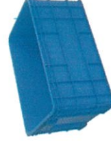
Model : 8069/2551/110 Ext. Size : 420 x 610 x 320 MM. Int. Size : 385 x 580 x 300 MM.
