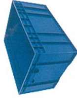
Model : C1130 Ext. Size : 470 x 640 x 330 MM. Int. Size : 450 x 550 x 360 MM.
