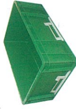
Model : 331 Ext. Size : 335 x 335 x 103 MM. Int. Size : 330 x 300 x 90 MM.
