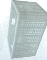
Model : 044V Ext. Size : 375 x 570 x 310 MM. Int. Size : 340 x 540 x 295 MM.
