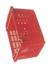
Model : 127N Ext. Size : 375 x 570 x 315 MM. Int. Size : 330 x 535 x 290 MM.
