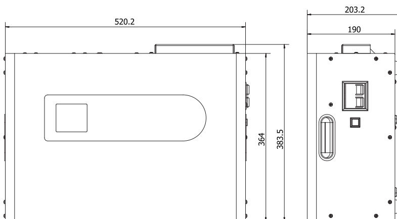
MST-20KVA
