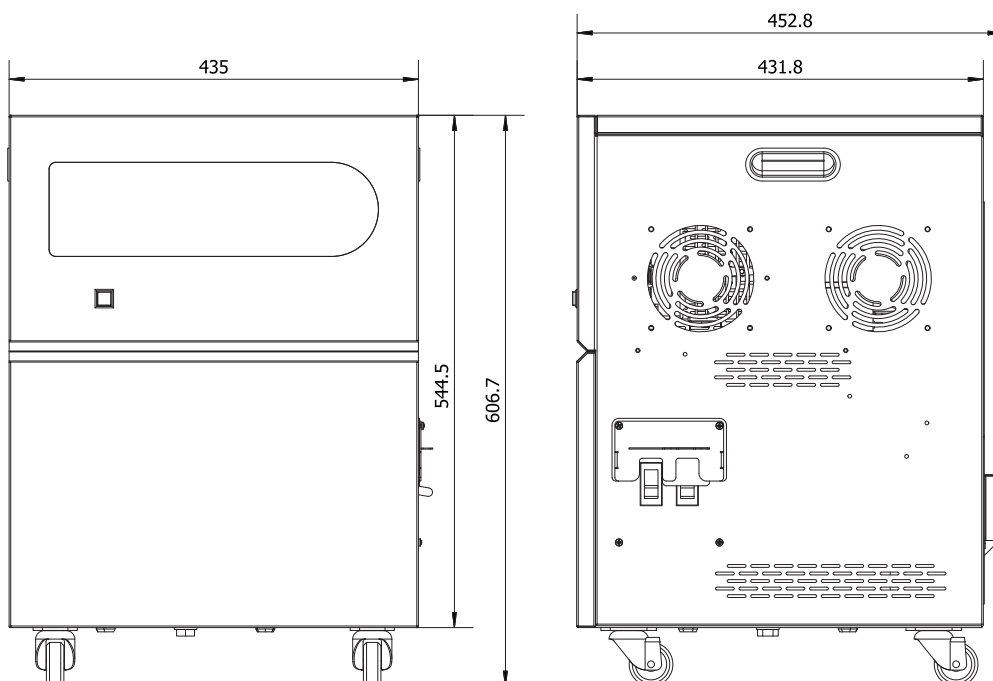
MST-30KVA
