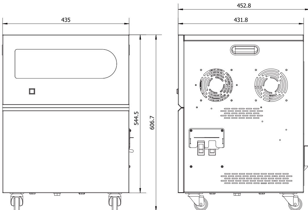
MST-30KVA
