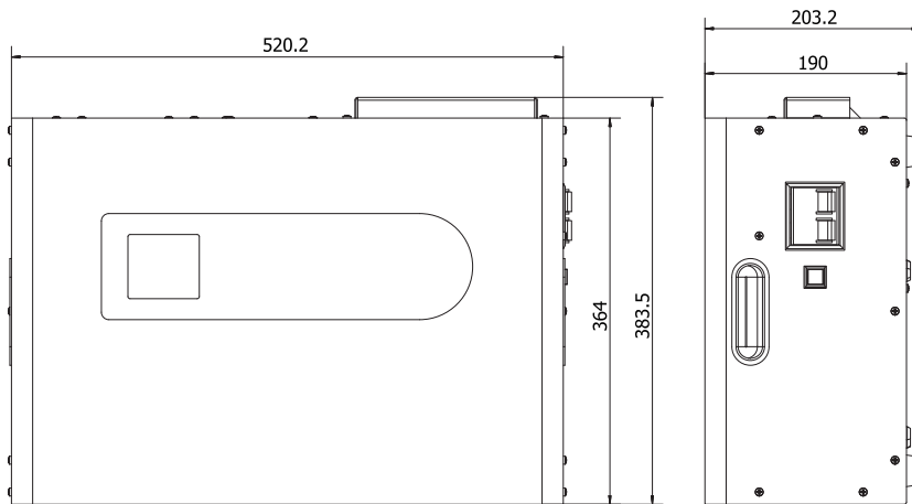
MST-20KVA
