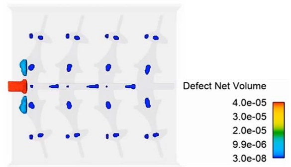
ปริมาณรูพรุนที่เกิดขึ้นหลังจากการแข็งตัว
