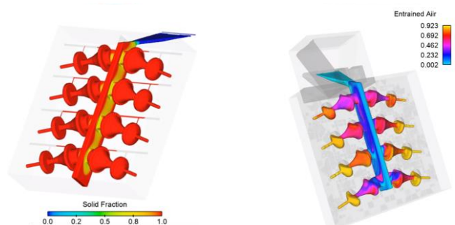
ปริมาณอากาศที่ปะปนในน้ำโลหะ
