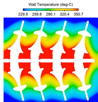
อุณหภูมิของแม่พิมพ์จากการวิเคราะห์
