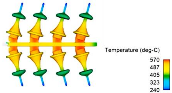
อุณหภูมิของน้ำโลหะขณะแข็งตัว
