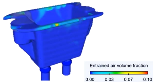
ปริมาณอากาศที่ปะปนในน้ำโลหะ
