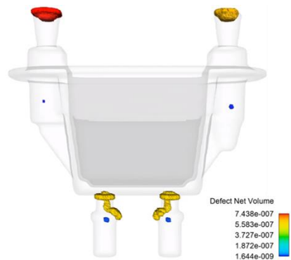
การวิเคราะห์ปริมาณรูพรุนที่เกิดขึ้นหลังการแข็งตัว
