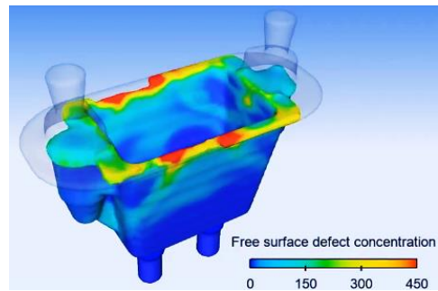
ปริมาณออกไซด์ที่ผิวหน้าโลหะ
