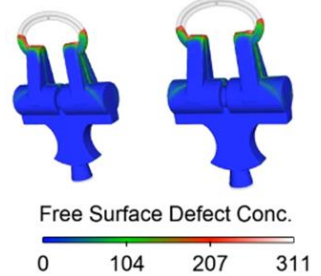
ปริมาณ Defect ที่ผิว น้ำโลหะ
