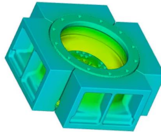
อุณหภูมิของแม่พิมพ์ขณะทำการผลิต
