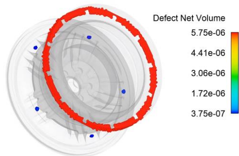
วิเคราะห์ปริมาณ Defect ที่เกิดขึ้นขณะแข็งตัว
