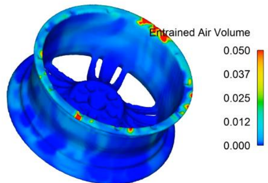
ปริมาณอากาศที่ปะปนในน้ำโลหะ
