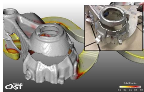
วิเคราะห์การเกิดการแข็งตัวก่อน (Early solidification)
