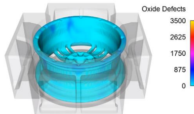
การเกิดออกไซด์ปะปนในน้ำโลหะ
