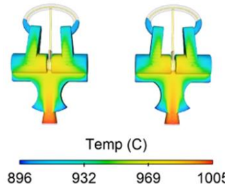
อุณหภูมิน้ำโลหะ
