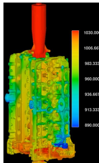
ความเร็วการไหลของน้ำโลหะ
