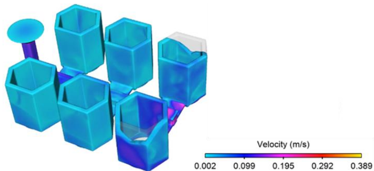
ความเร็วการไหลของน้ำโลหะ
