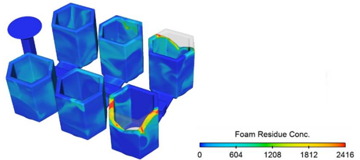
การวิเคราะห์ปริมาณโฟมที่ตกค้างและปะปนในน้ำโลหะ
