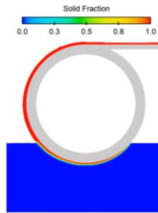
สัดส่วนของแข็งในการหล่อแบบ Continuous sheet casting
