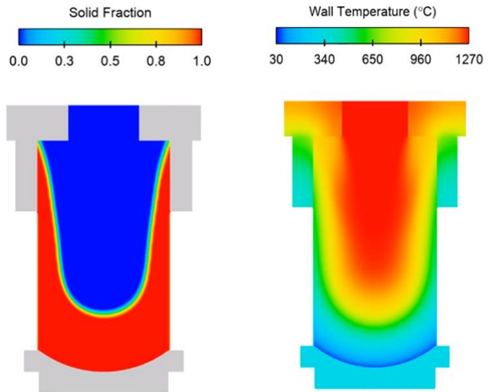
วิเคราะห์สัดส่วนของแข็งในงาน
