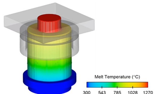
อุณหภูมิของโลหะขณะทำการหล่อแบบ Direct chill casting
