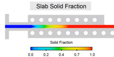
สัดส่วนของแข็งของการหล่อ Slab
