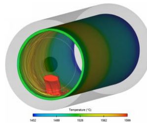
งานหล่อเหวี่ยงท่อนในแนวนอน
