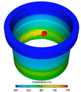
งานหล่อเหวี่ยงในแนวตั้ง
