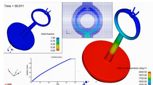
วิเคราะห์การเกิดโพรงหดตัว (Shrinkage porosity)
