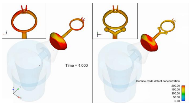
การเกิดออกไซด์ในน้ำโลหะ
