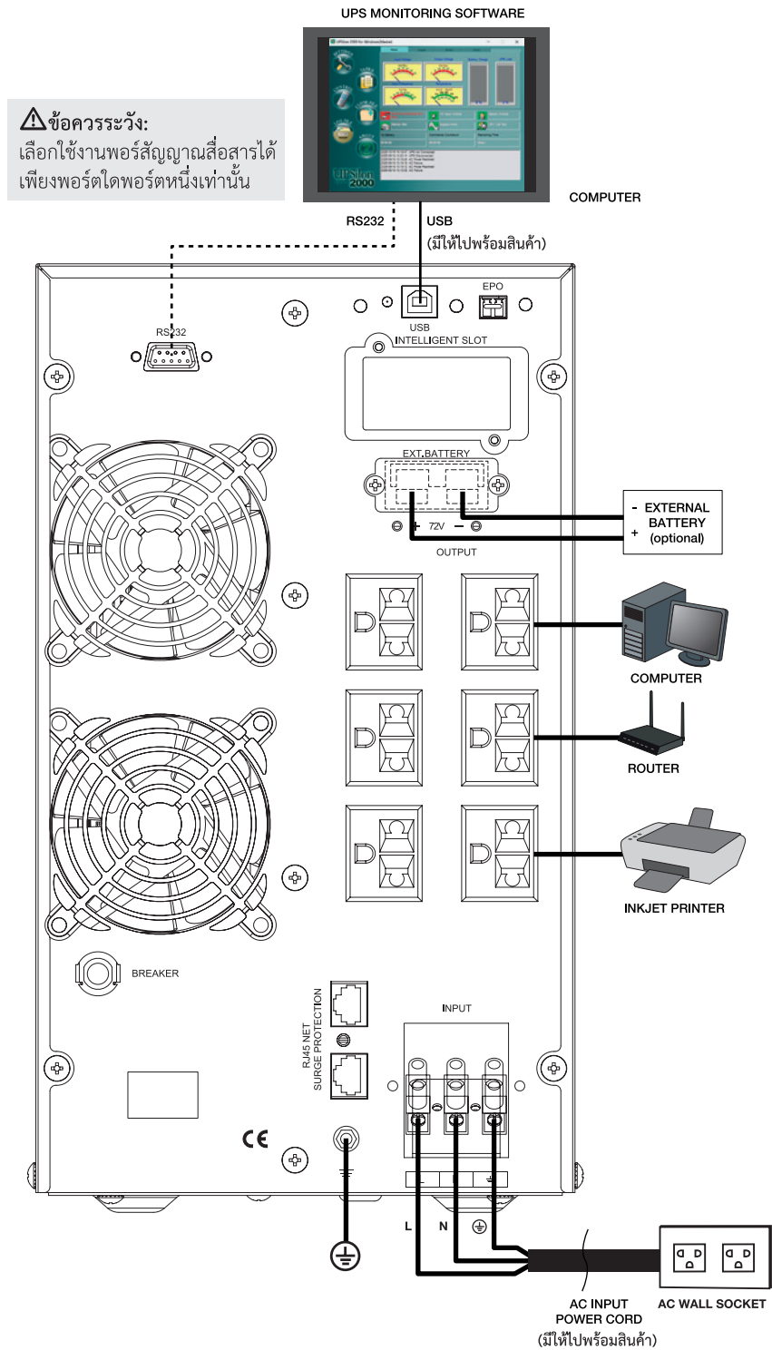
ภาพตัวอย่างการติดตั้งในรุ่น UKA-4K
