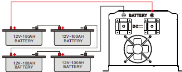
การเชื่อมต่อแบตเตอรี่ระบบ 48V
