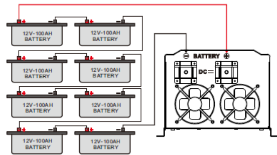
การเชื่อมต่อแบตเตอรี่ระบบ 96V
