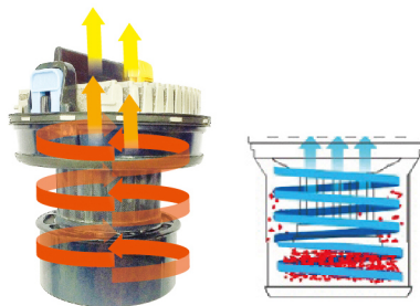
การแยกฝุ่นระบบพลังหมุน
