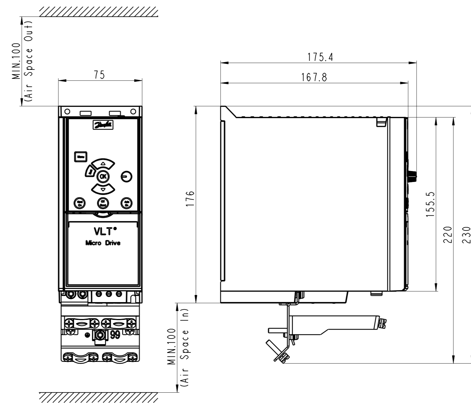
DECOUPLING-OPTION
