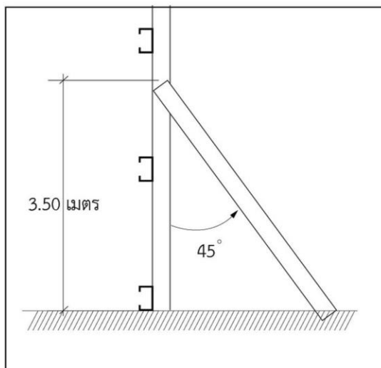
ภาพแสดง รายละเอียดระยะขาตั้งโครงสร้าง
