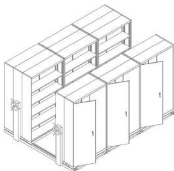
CPT-305 (3 แถว) 2540(L) x 3660(W) x 2250(H) mm.
