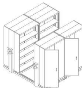
CPT-205 (2 แถว) 2540(L) x 2440(W) x 2250(H) mm.
