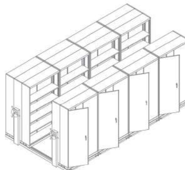
CPT-405 (4 แถว) 2540(L) x 4880(W) x 2250(H) mm.
