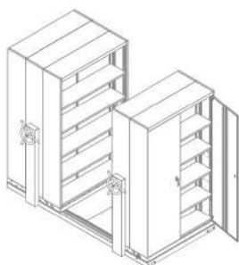
CPT-105 (1 แถว) 2540(L) x 1220(W) x 2250(H) mm.
