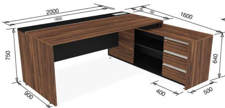
2EX2016R R/L (แผ่น TOP 2-TONE) 2000(W) x 1600(D) x 750(H) mm.
