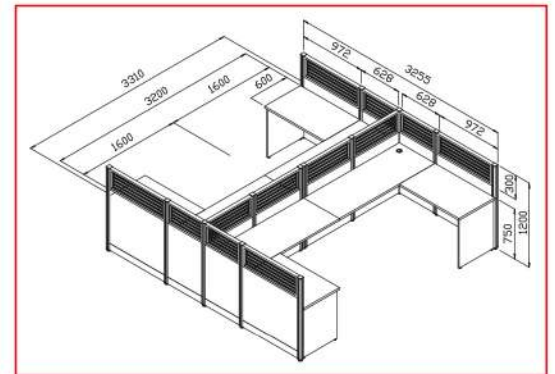
MT-WS024 (ชุด workstation 4 ที่นั่ง) 3310(W) x 3255(D) x 1200(H) mm.
