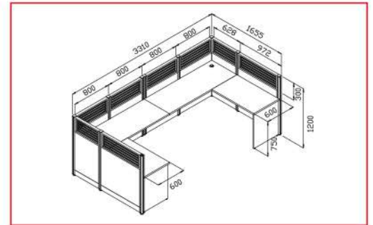
MT-WS022 (ชุด workstation 2 ที่นั่ง) 3310(W) x 1655(D) x 1200(H) mm.
